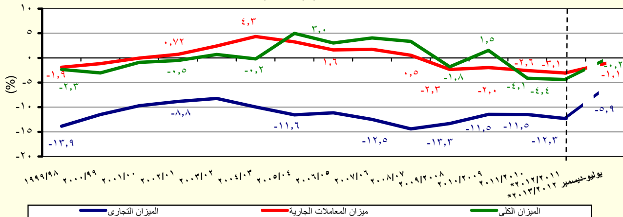
شكل (٢٤): مؤشرات مختارة لمعاملات القطاع الخارجي (نسبة إلى الناتج المحلي الإجمالي)
